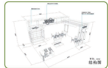
展台内部钢结构图:
